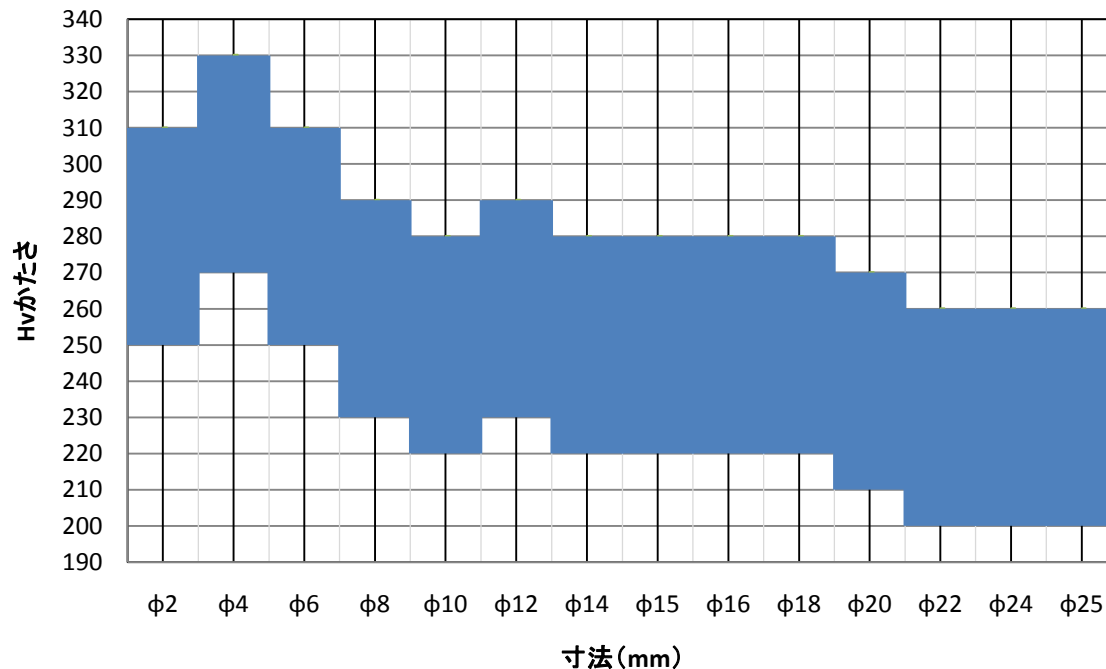
SUS304-D 寸法別機械的性質:Hvかたさ(中心)
