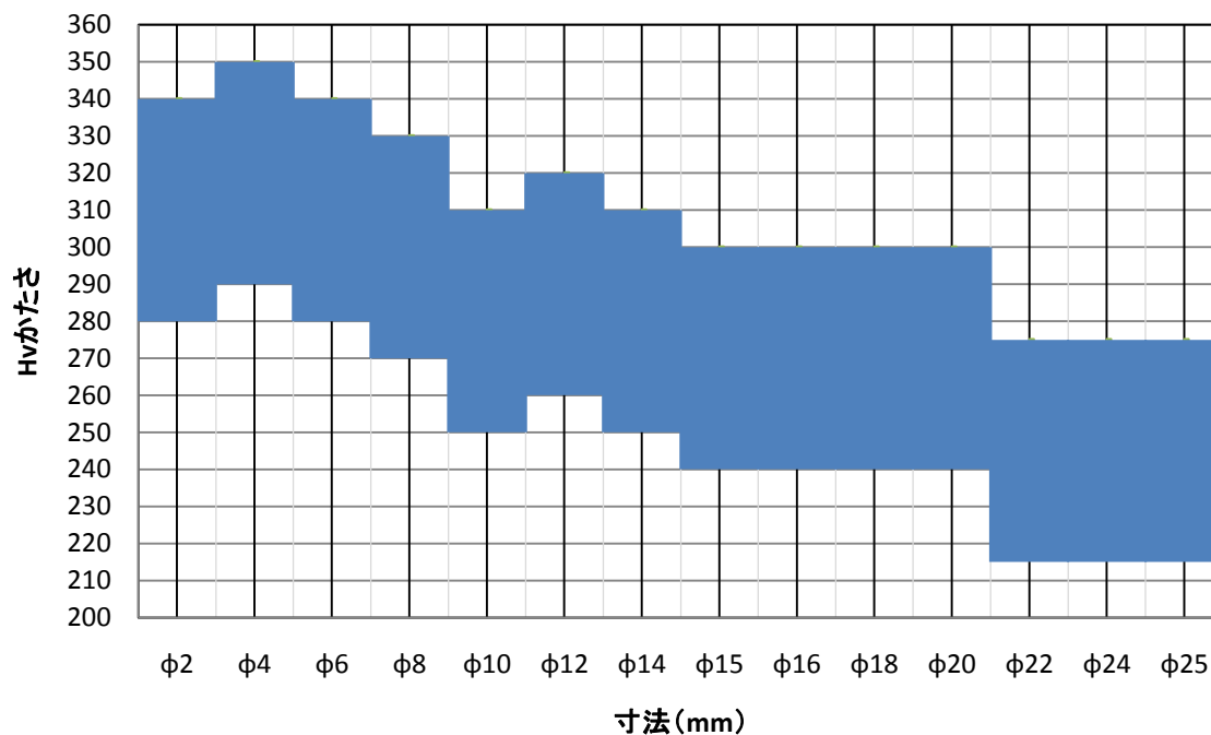
SUS304-D 寸法別機械的性質:Hvかたさ(測定位置:直径/4)
