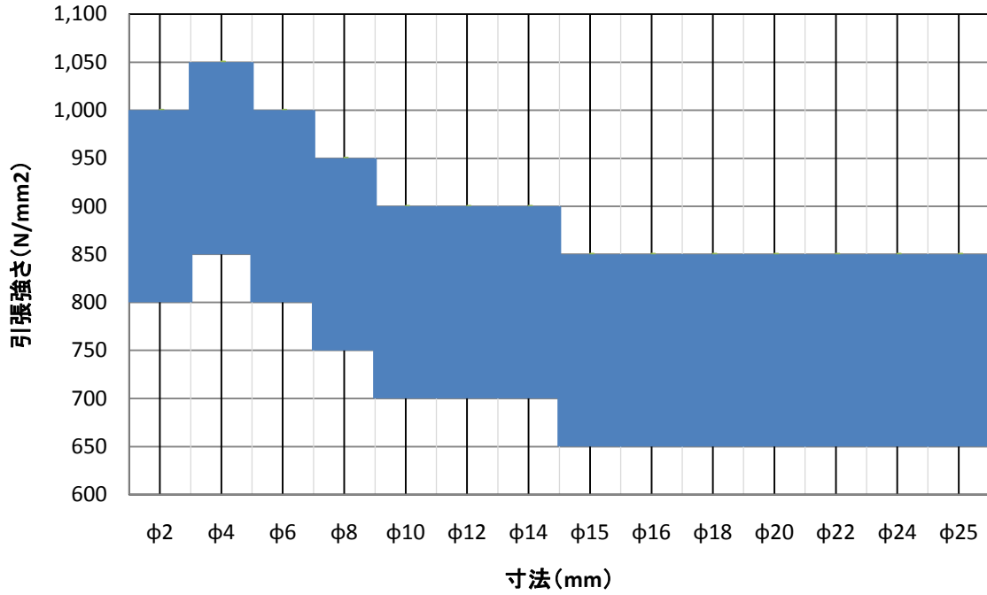
SUS304-D 寸法別機械的性質:引張強さ
