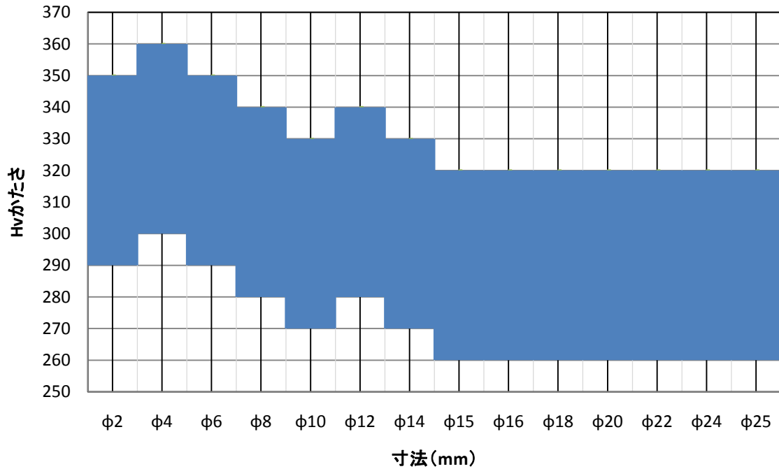
SUS304-D 寸法別機械的性質:Hvかたさ(測定位置:表層部)
