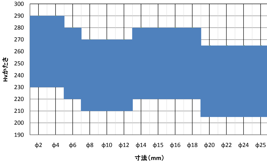
SF20T・SF20F 寸法別機械的性質:Hvかたさ
