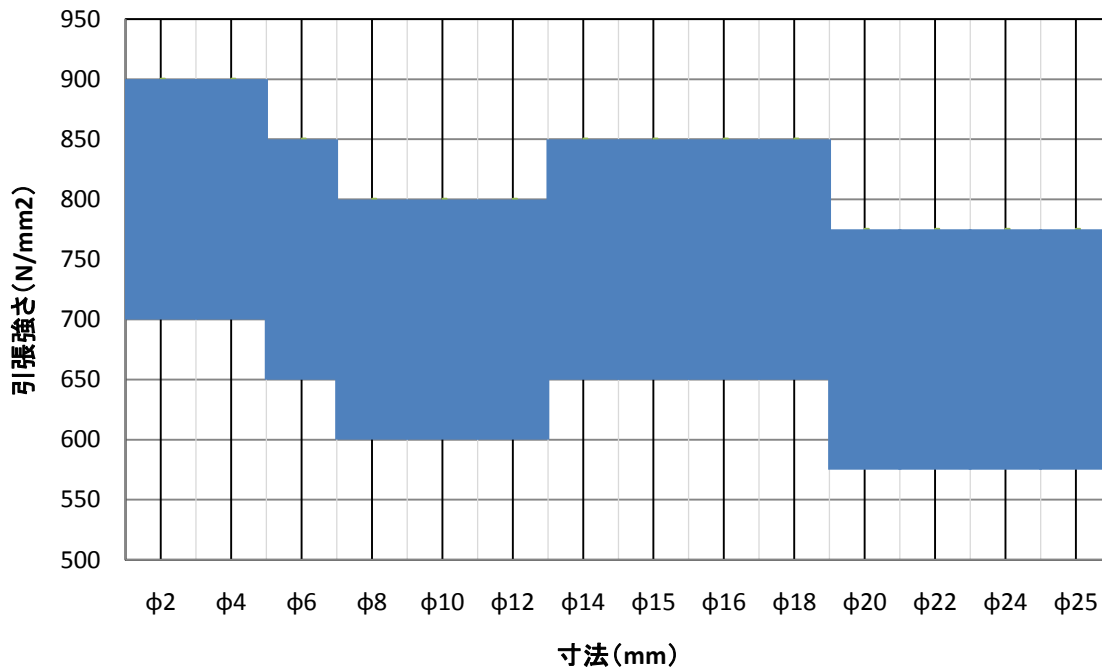
SF20T・SF20F 寸法別機械的性質:引張強さ
